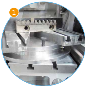
1) Sonderspanneinrichtung 2) Seitliche Durchführung links oder rechts
