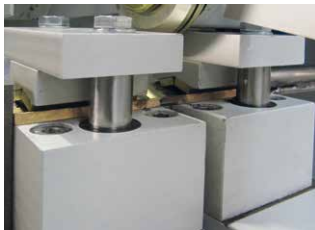
Spannung von 10 bis 20 mm mit wechselbaren Aufnahmen
