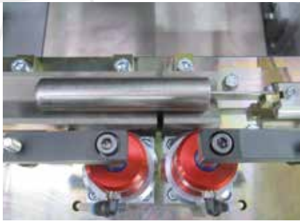
Prismenspannung mit zwei pneumatischen Schwenkspannern und digitalem Werkstückanschlag.
