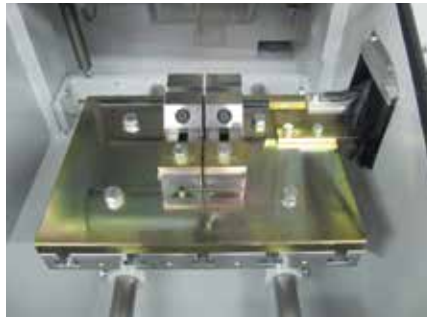
Parallelspannstücke für Materialgröße 2-20 mm mit digitalem Werkstückanschlag.
